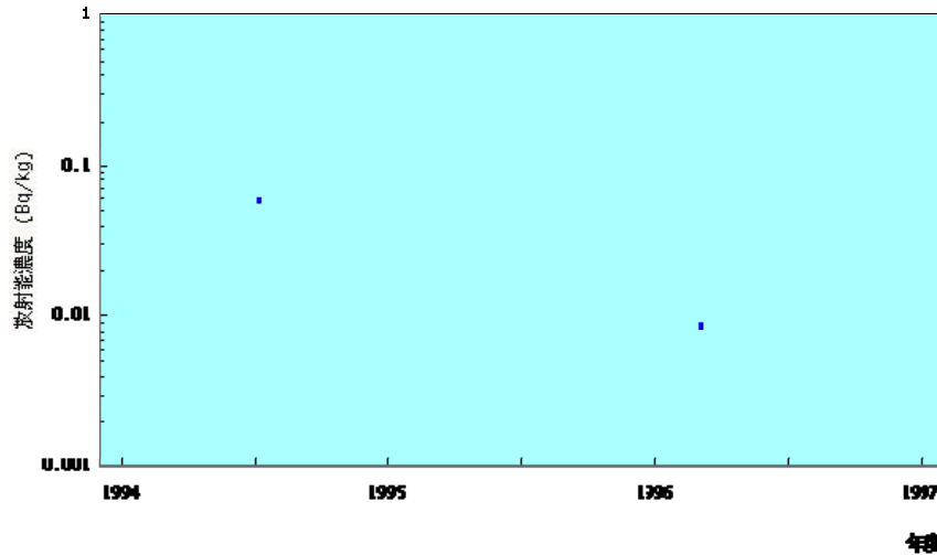
北陸・甲信越地方におけるメロン中のCs-137の経年変化
